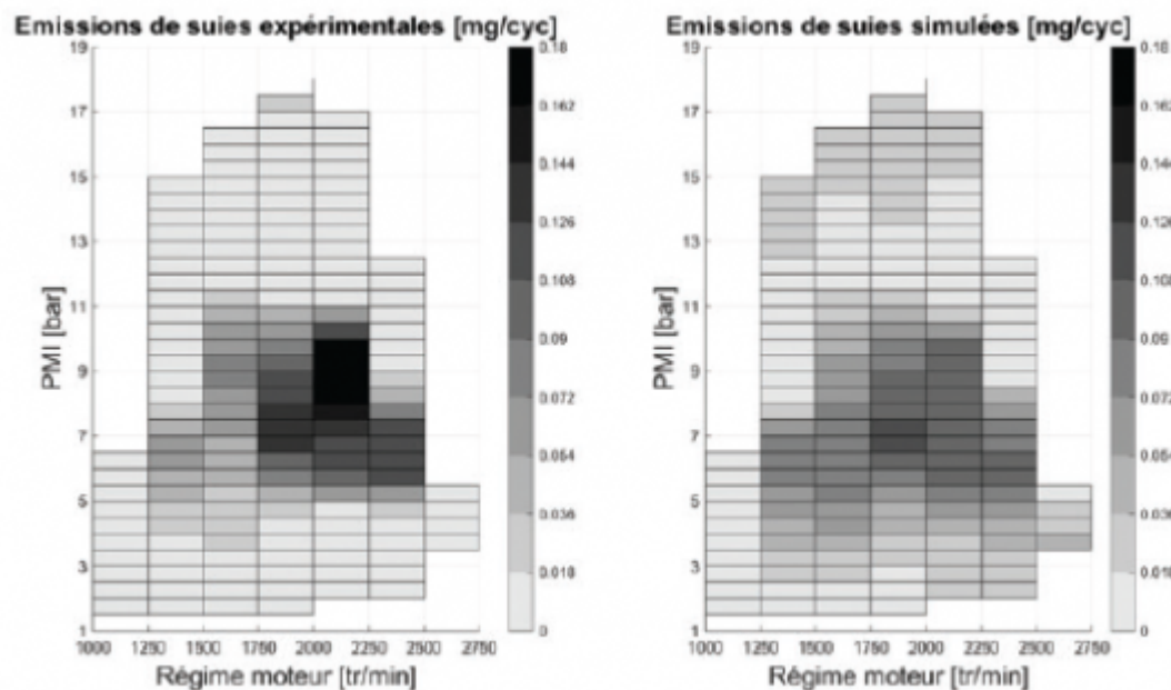
Comparaison des quantités de suies mesurées et calculées dans le domaine de fonctionnement du moteur[b].
