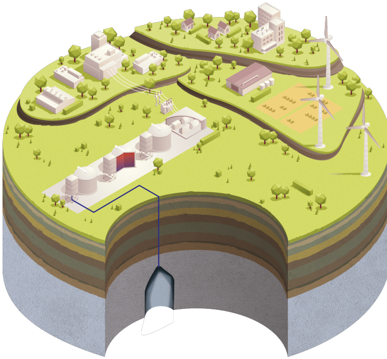
Stockage Energie par Air Comprimé - Adiabatique Avancé
