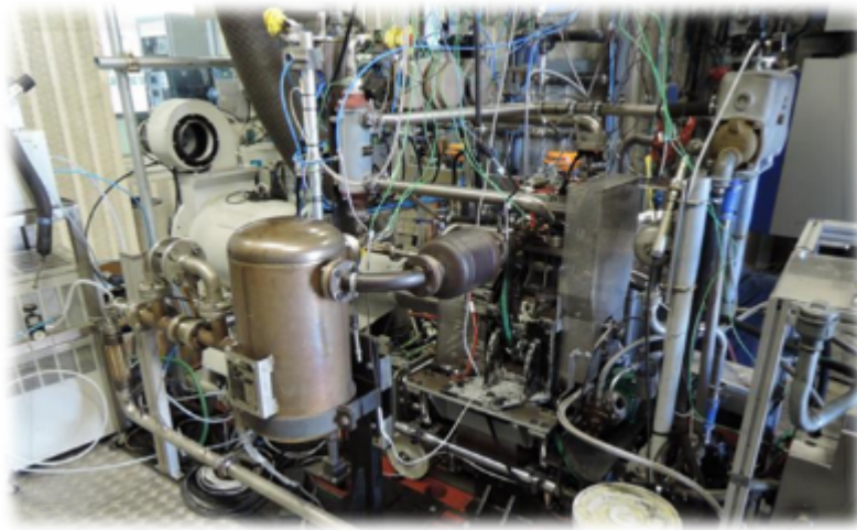
Banc H2 monocylinde véhicule léger
