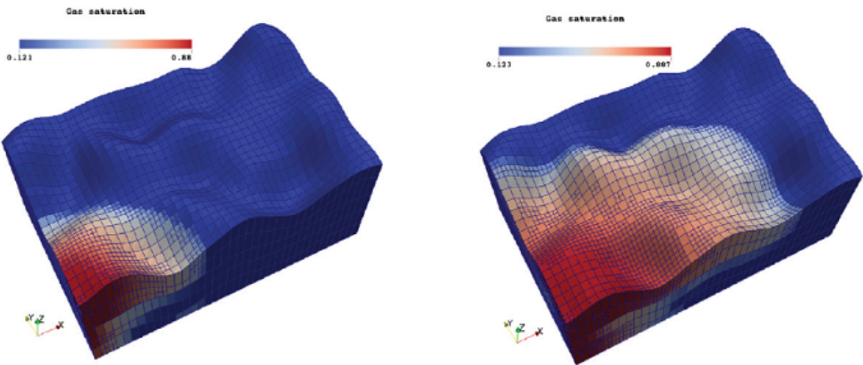
Résultat à 500 et 1 500 jours d'un calcul d'écoulement multiphasique, utilisant un maillage adaptatif.
